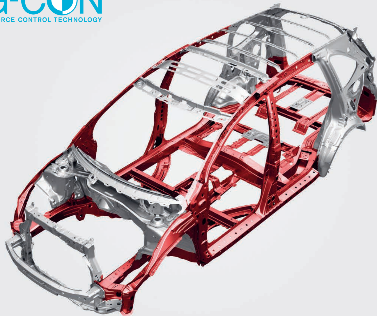
Estructura de carrocería con Ingeniería de Compatibilidad Avanzada (ACE®) II.
